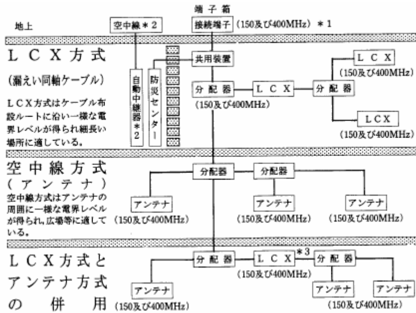
別図 無線通信補助設備の方式
