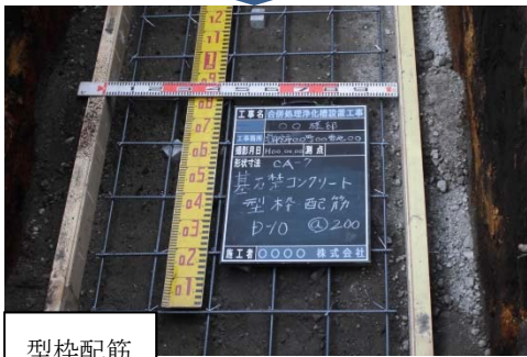
型枠配筋
