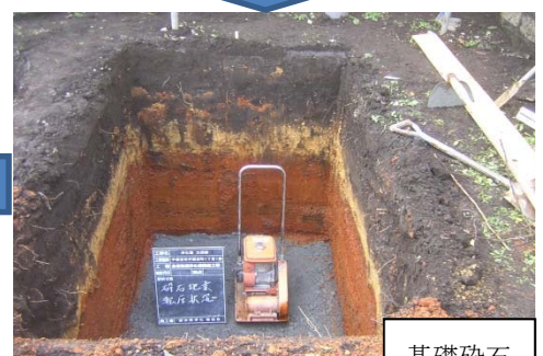
基礎碎石
