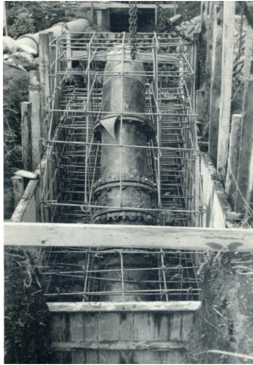
布設中の配水管（奈坪川水管橋）
