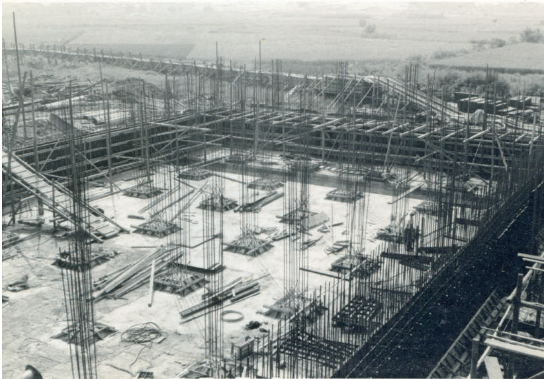
建築中の白沢水源地ポンプ室兼事務所(昭和43年)
