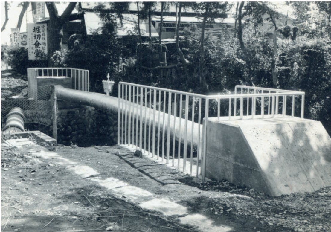
完成した配水管（奈坪川水管橋）
