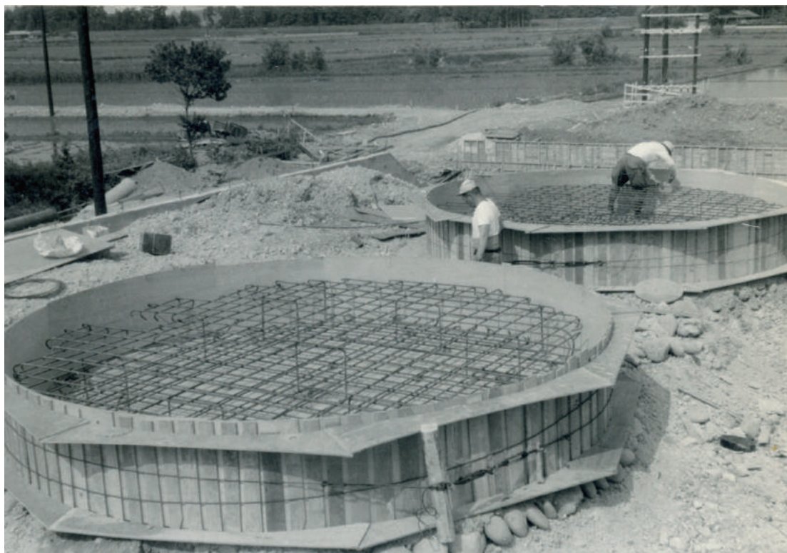
白沢水源地1・2号取水井構造工事(昭和43年度)
