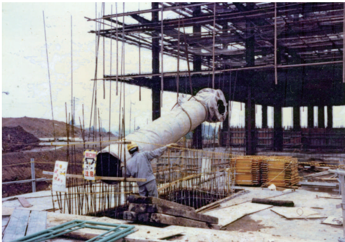
管理棟本館工事 (昭和53年4月)
